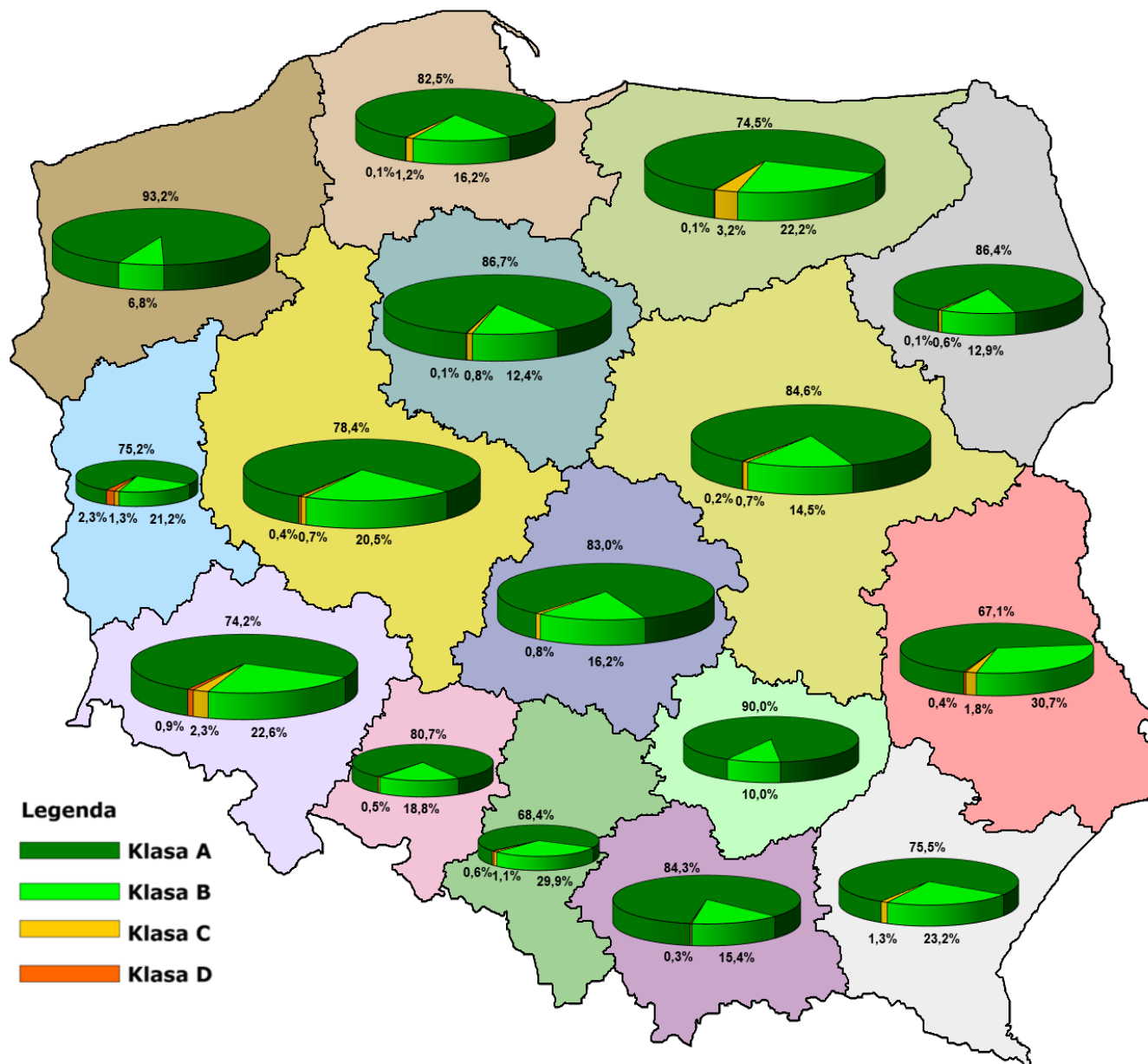
Rysunek 6. Stan techniczny pod względem parametru: równość podłużna
